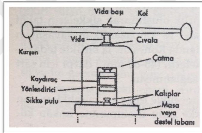
Çizim 4: Sikke basma makinesi,
