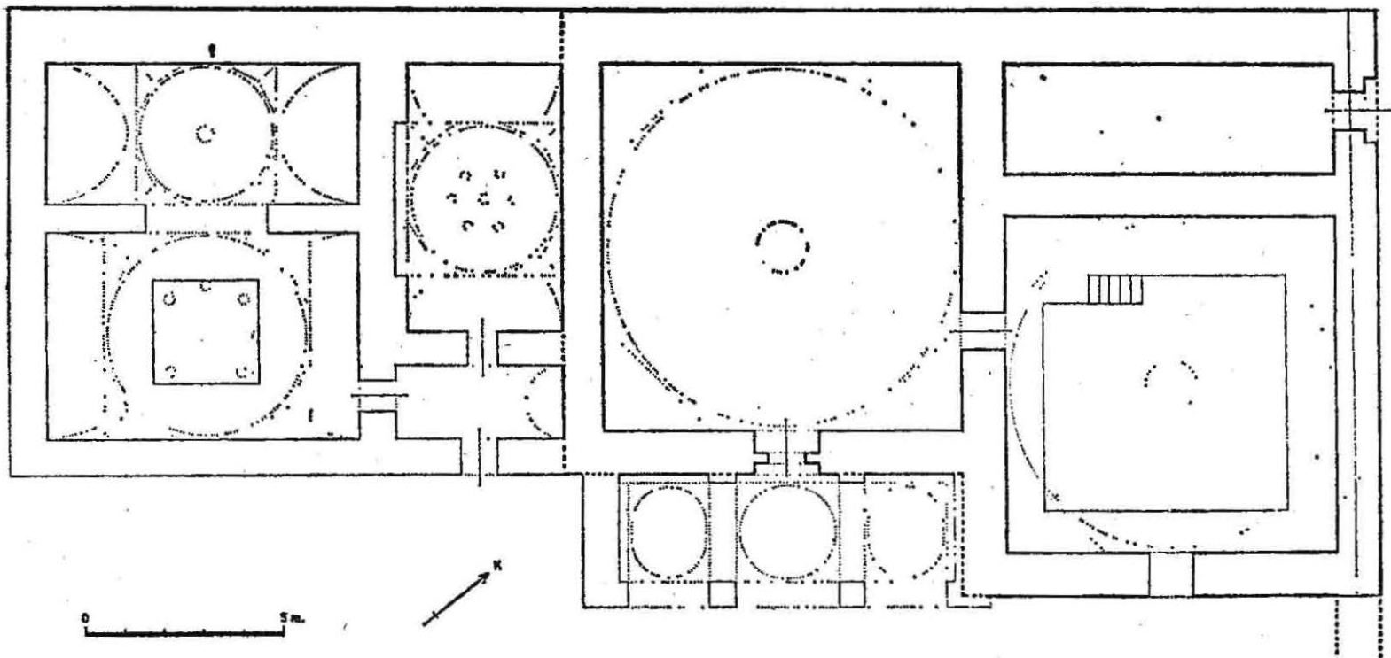
Plân III - Y. Müh. Mimar Prof. Dr. Yılmaz Önge tarafından, Vakıflar Genel Müdürlüğü Arşivindeki projesinden tādilen çizilen plân.
