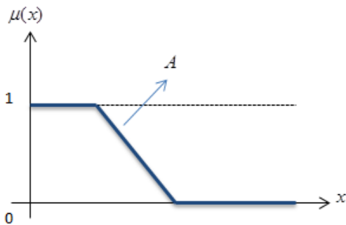
Şekil 1.1.1.6. A bulanık kümesi
