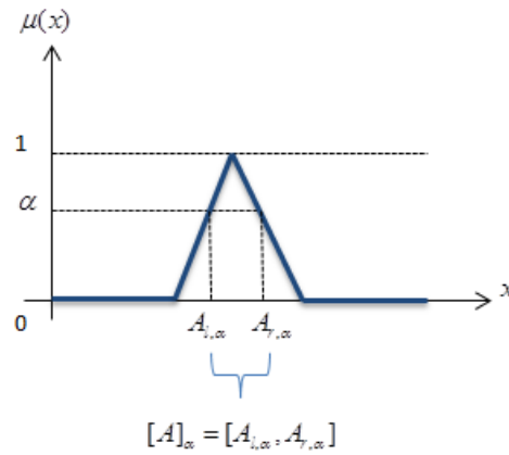
Şekil 1.1.1.8. A bulanık kümesinin \alpha -kesimi
