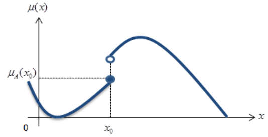
Şekil 1.1.1.13. Üst-yarı sürekli değil (Alt-yarı sürekli)
