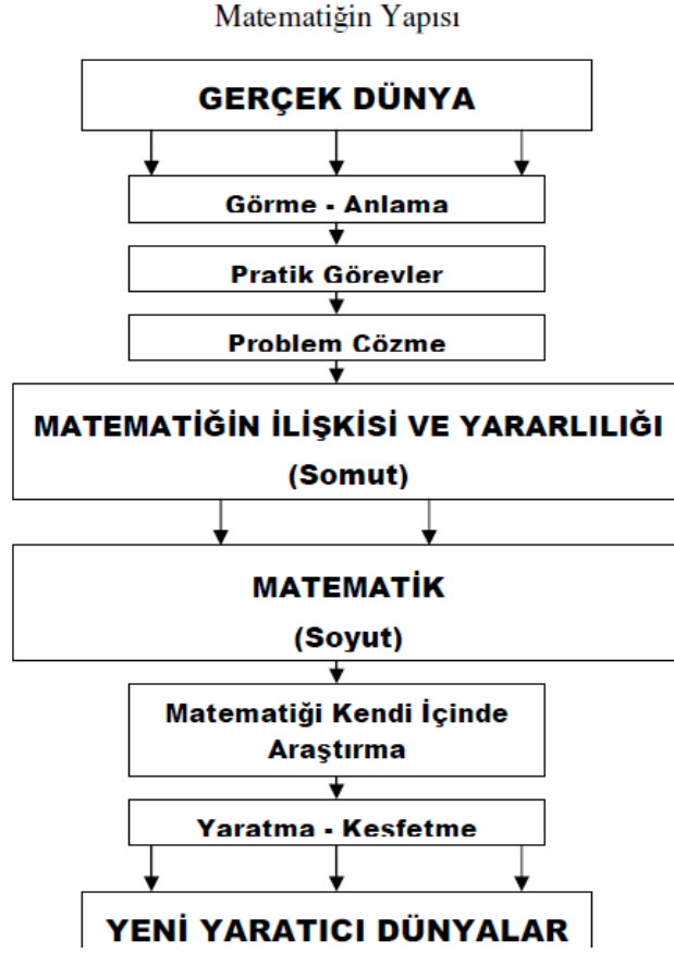
Şekil 2: Matematiğin Yapısı
