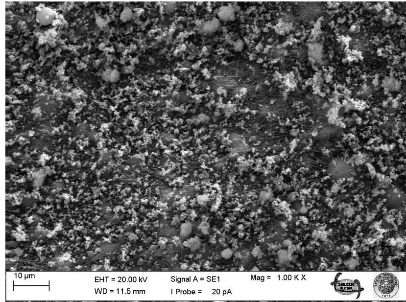
Şekil 3. Dördüncü nanofiber filtrenin (3,2 g/m 2 ) morfolojisi ve yakaladığı CaCO 3 nanopartiküller Figure 3. Morphology of fourth nanofiber filter (3,2 g/m 2 ) and captured CaCO 3 nanoparticles
