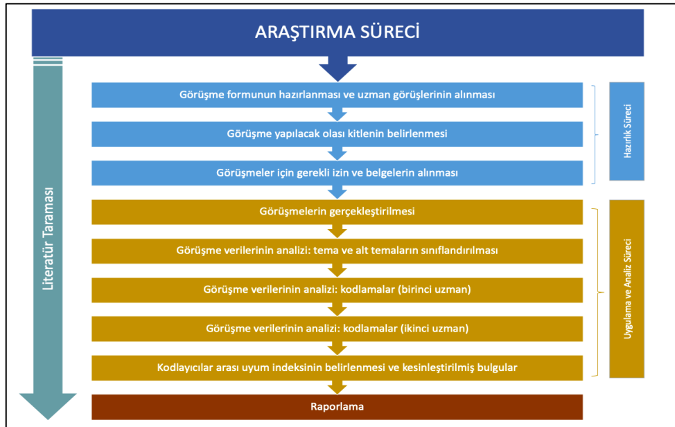
Şekil 2. 1. Araştırma Süreci
