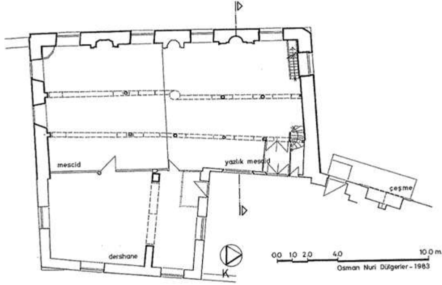
Çizim 3. 5: Hoca Mahmud, Mektep, Cami ve Türbesi Planı (O.N. Dülgerler'den)
