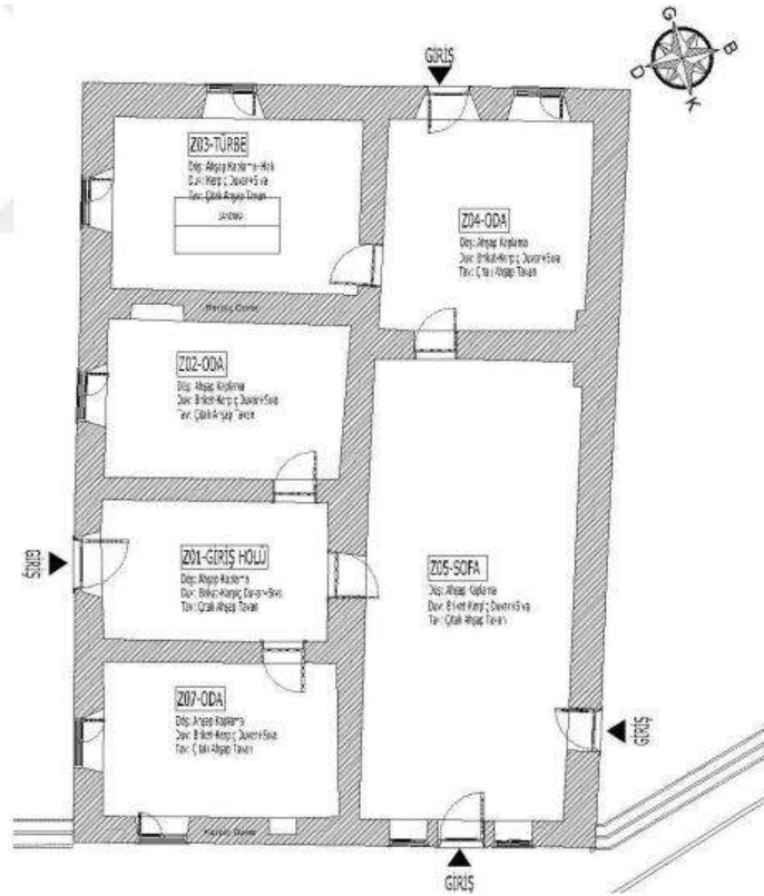
Çizim 3. 1: Ebü İshak Kâzerûnî Zaviyesi Planı (Toydemir, 2022)
