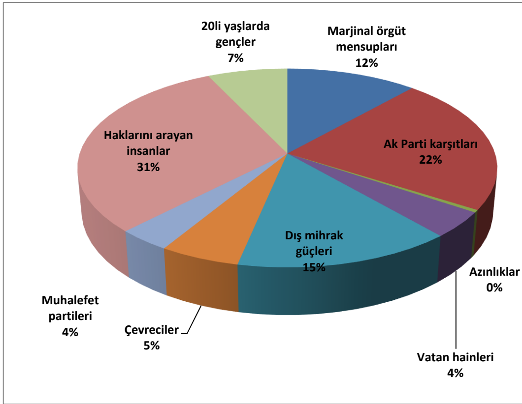
Şekil 3.7.1.13. Eylemcileri Tanımlama
