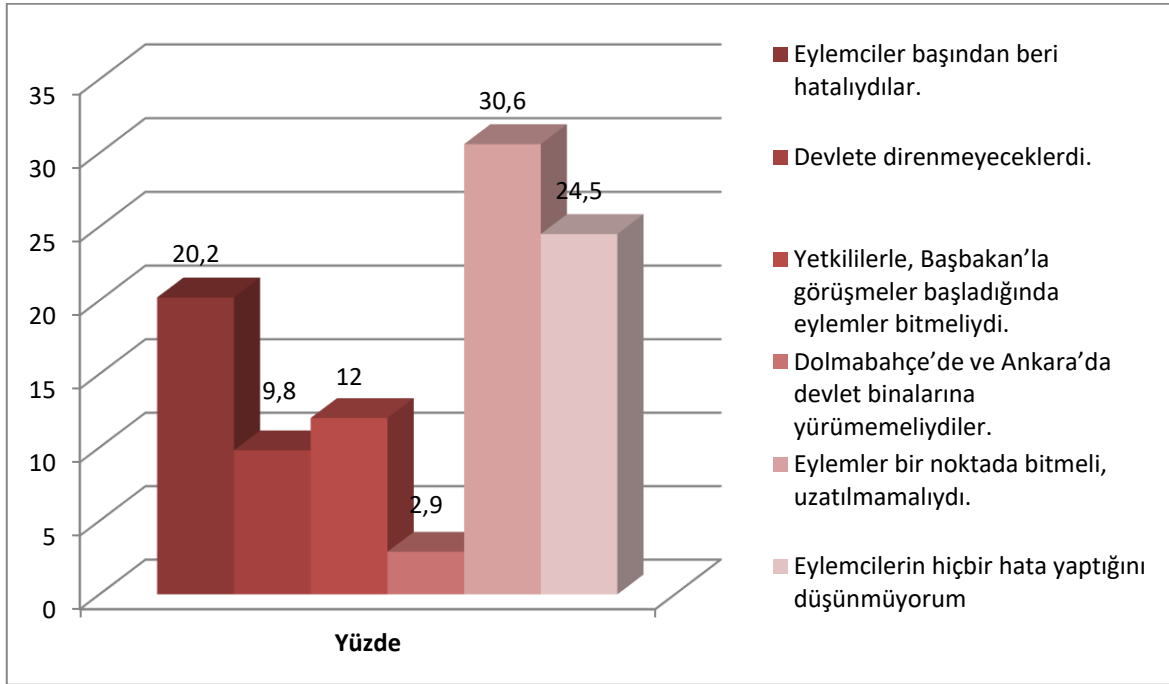
Şekil 3.7.1.10. Eylemcilerin Değerlendirilmesi
