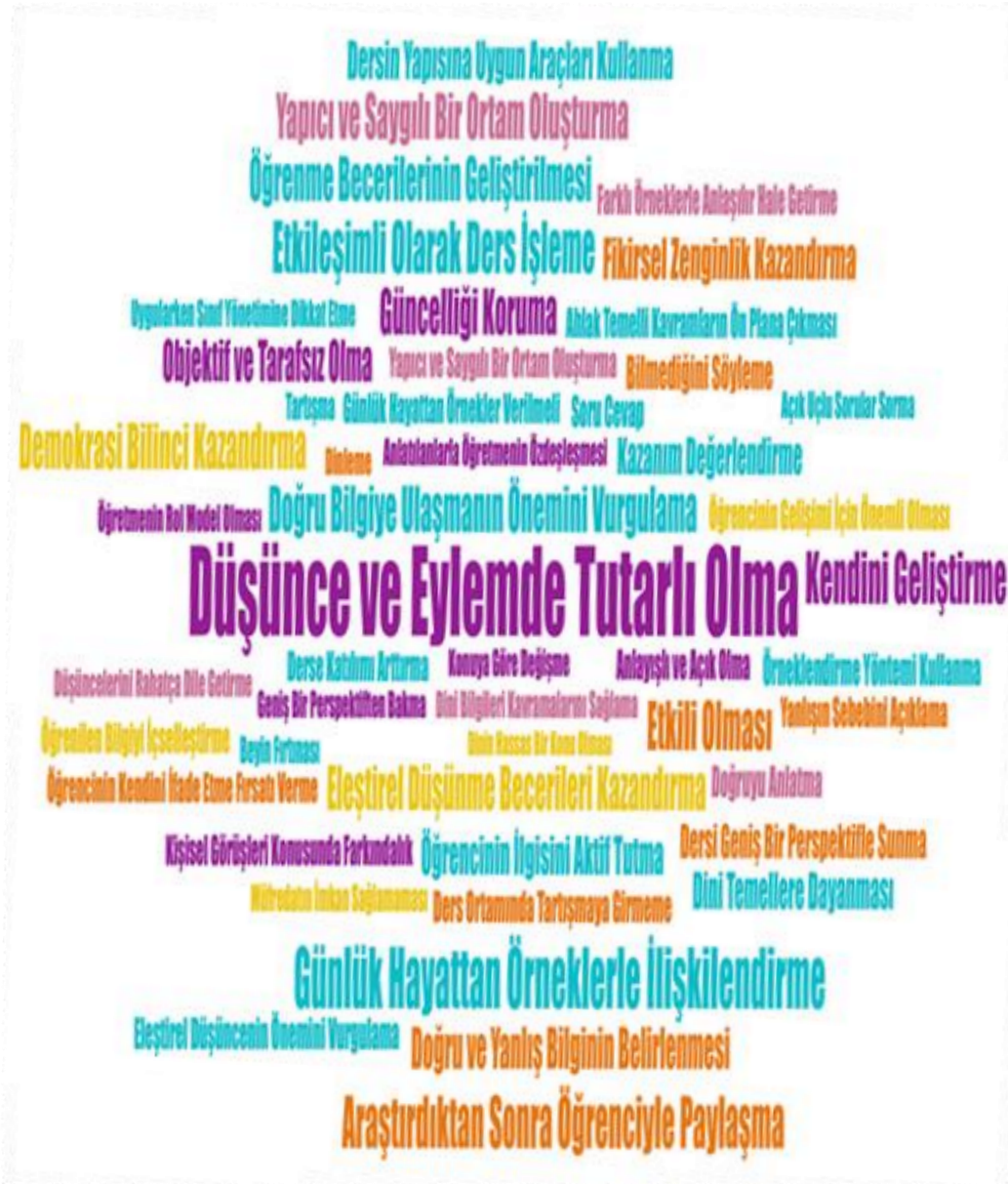
Şekil 3.12. Kod Bulutu
