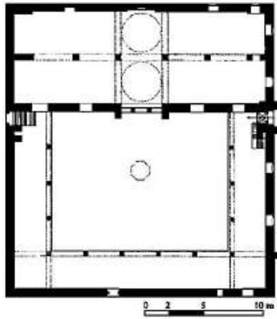
Plân: 3 Selçuk İsa Bey Camii plânı (S. Eroğlu'dan)
