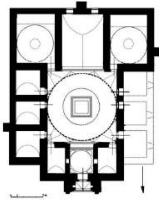
Plân: 7 Kütahya Vâcidiye Medresesi plânı (S. Eroğlu'dan)
