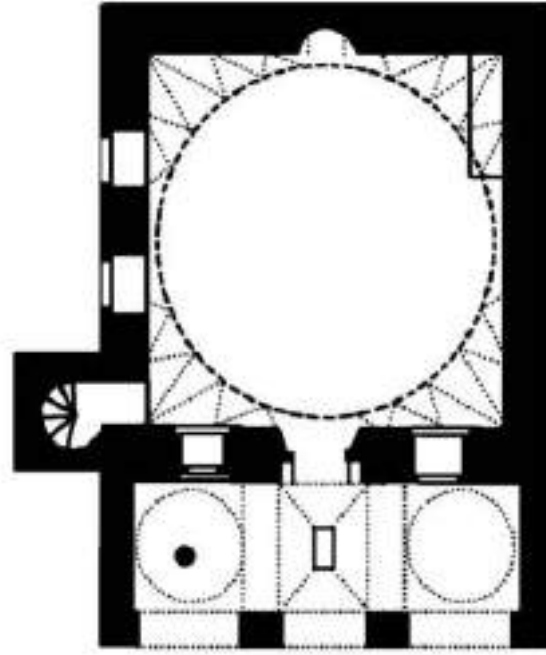
Plân: 6 Kütahya Kurşunlu Camii plânı (S. Eroğlu'dan)
