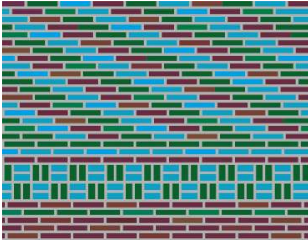
Çizim: 31 Minare gövdesinin sırlı tuğla yerleşimi
