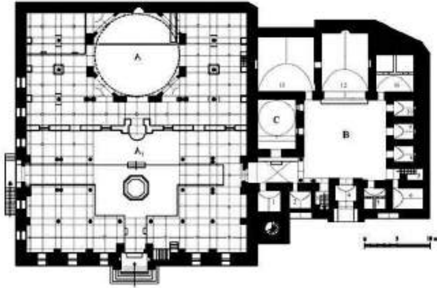
Plân: 9 Manisa Ulu Camii plânı (S. Eroğlu'dan)
