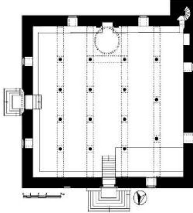
Plân:1 Birgi Ulu Camii plânı (S. Eroğlu'dan)
