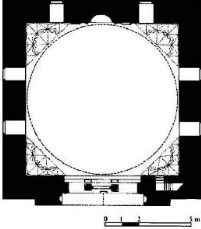
Plân: 8 Balat İlyas Bey Camii plânı (S. Eroğlu'dan)
