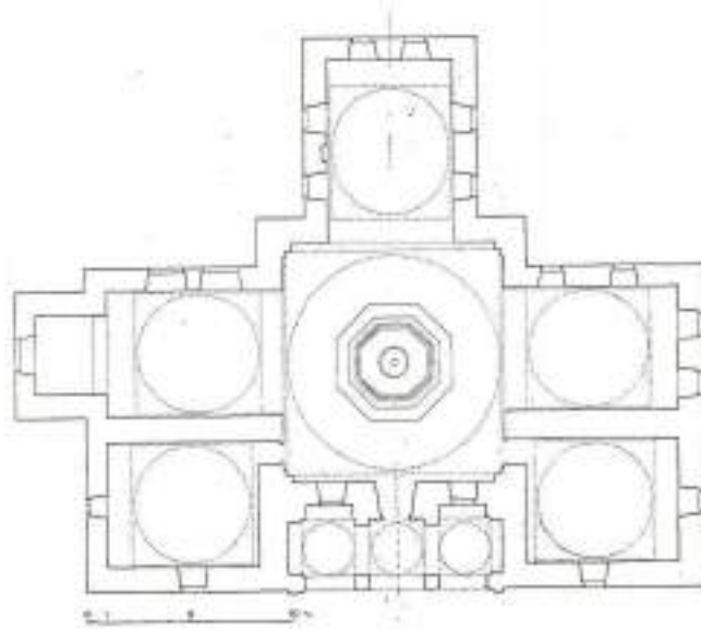
Plân: 4 Kütahya II. Yakup Bey İmareti plânı (A. Kızıltan'dan)
