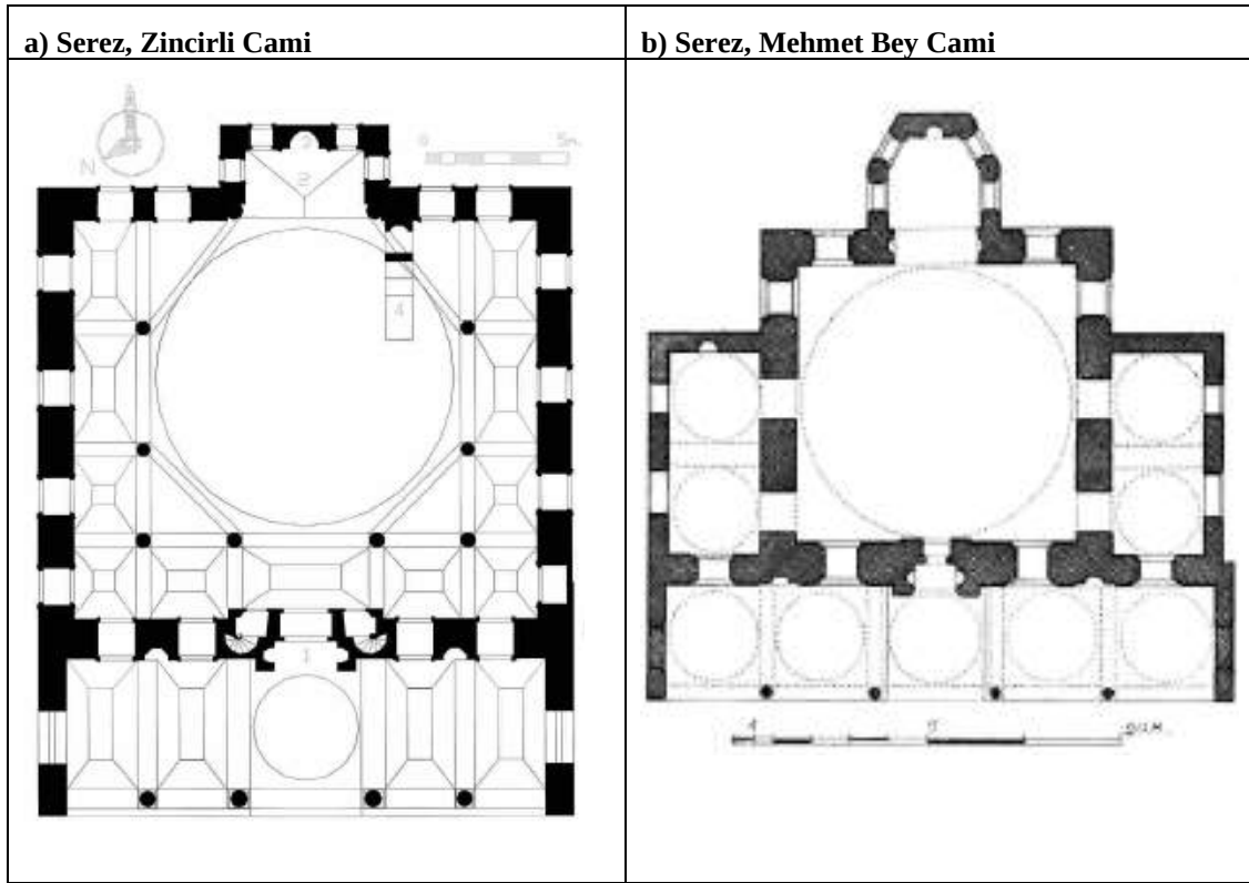
Plan 9. Zincirli Cami planı (Ameen, 2017), Mehmet Bey Cami planı (Anhegger, 1967).
