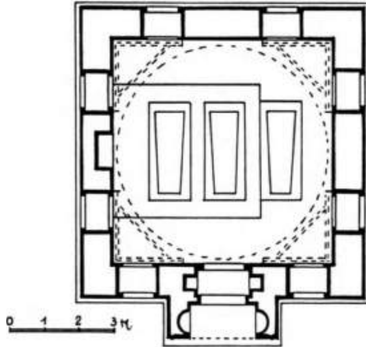
Plan 12. Mükrim Hatun Türbesi (Şah Sultan Türbesi) planı (Önkal, 1992).
