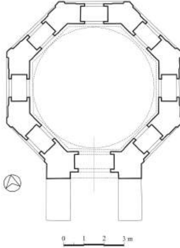
Plan 3. Selçuk Sultan Türbesi Planı (Doğanay, 2001).
