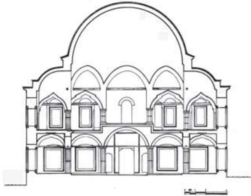
Plan 7. Zincirli Cami enine kesit kuzeydoğu (Brouskari, 2008).
