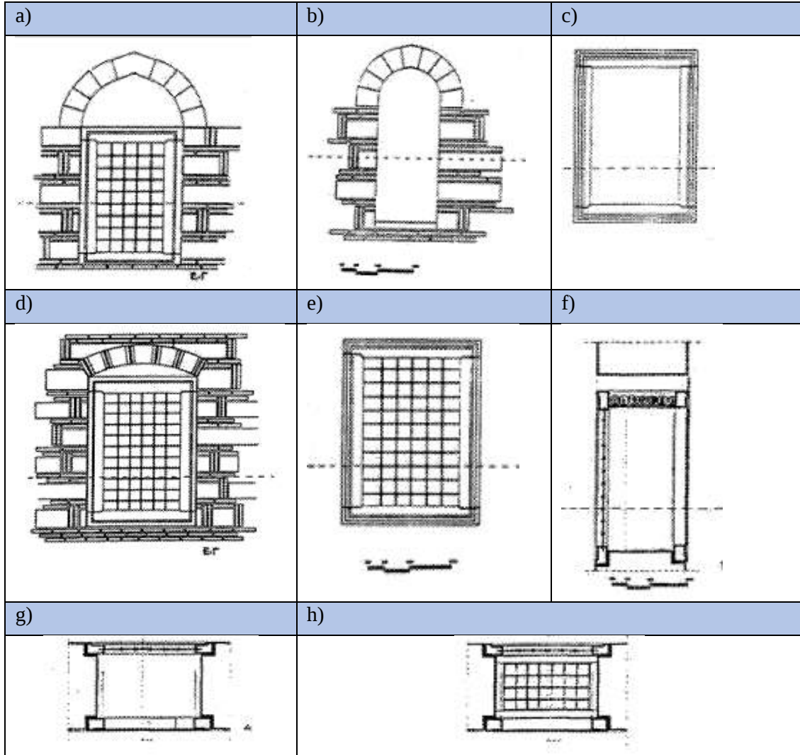
Çizim 1. Zincirli Cami pencere tipleri (Gavra, 1986).
