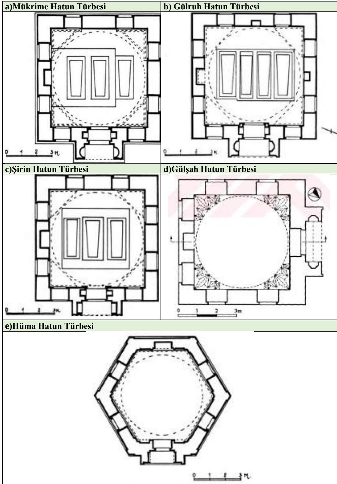
Plan 13. Mükrime Hatun, Gülrüh Hatun, Şirin Hatun, Gülşah Hatun, Hüma Hatun Türbeleri planları (Önkal, 1992 ve Daş, 2003).
