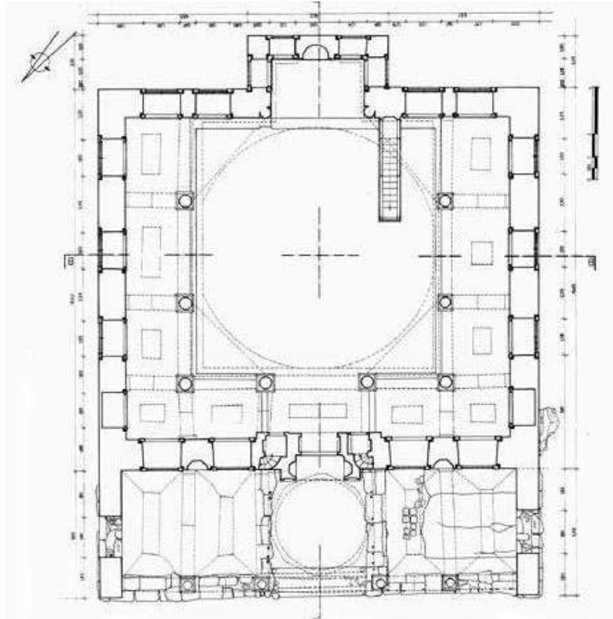
Plan 6. Zincirli Cami zemin kat planı (Bakirtzis ve Sambanopoulou, 2009).
