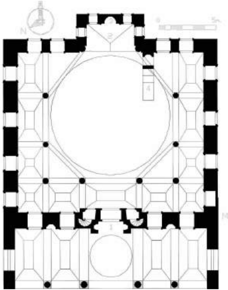
Plan 5. Zincirli Cami Planı (Ameen, 2017).
