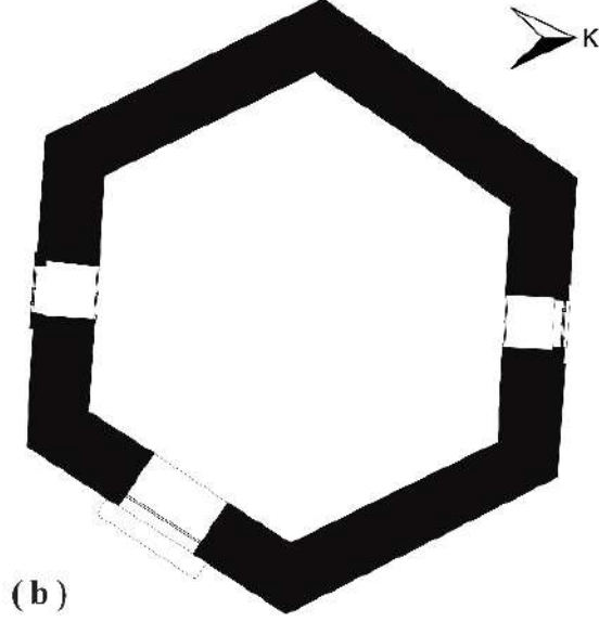
Çizim: 11: Kayabey Camii Müştemilatında Bulunan Üçpınarlıoğlu Türbe Planı 280
