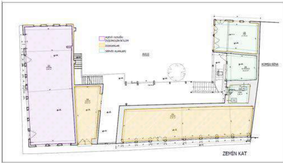
Çizim: 8: İmaret Medresesi zemin kat planı (Filiz Karakuş'tan)
