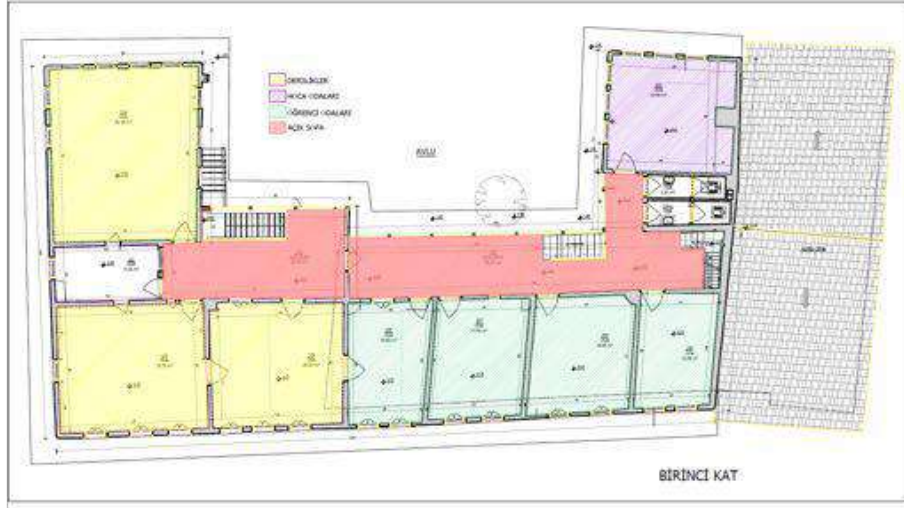
Çizim: 9: İmaret Medresesi birinci kat planı (Filiz Karakuş'tan)
