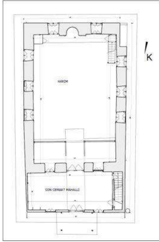
Çizim: 5: Mevcut Kasım Bey İmaret Camii Plan 264
