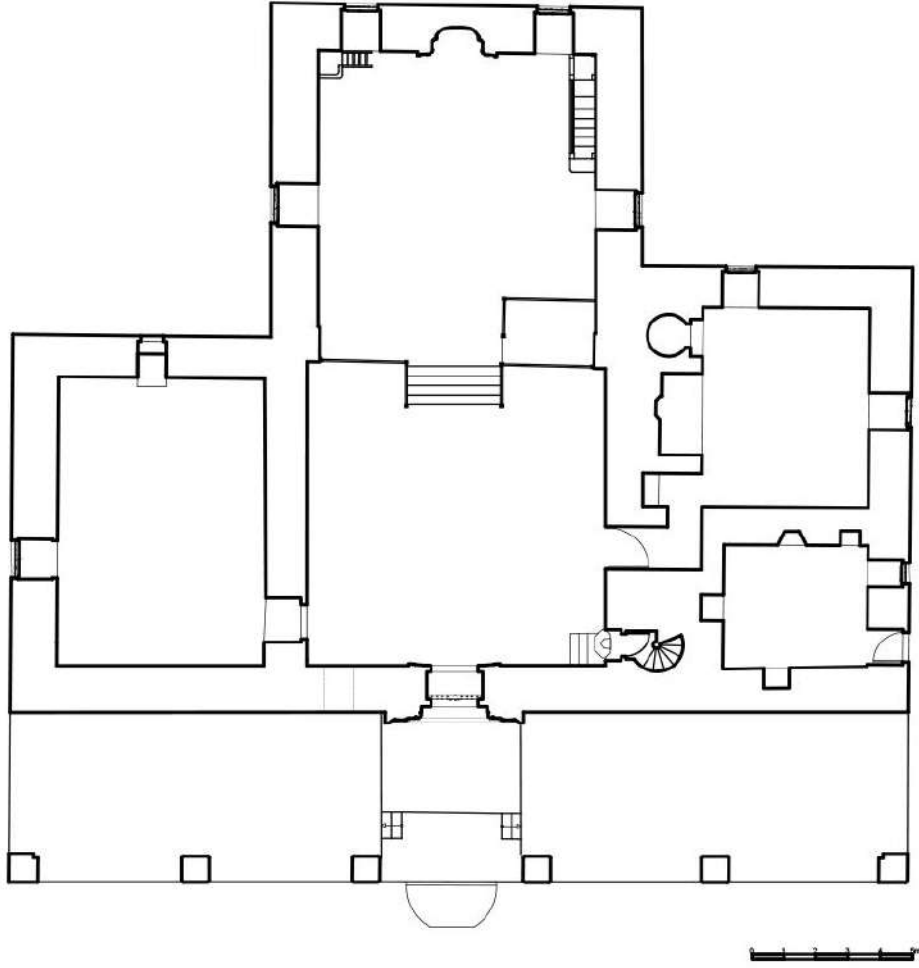
Çizim: 2: İsmail Bey Camii'nin Zemin Kat Planı 210
