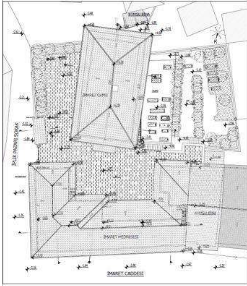
Çizim: 4: Mevcut Kasım Bey İmaret Vaziyet Planı 258
