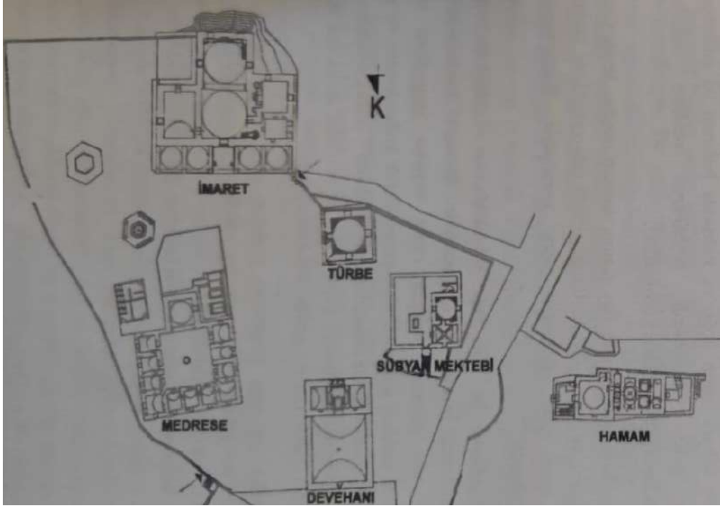
Çizim: 3:İmaret Vaziyet planı 217
