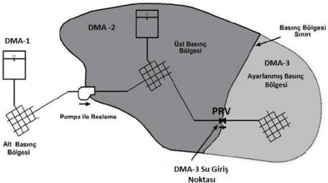
Şekil 2.5. DMA'larda PRV ile basınç yönetimi (Cinal, 2009)
