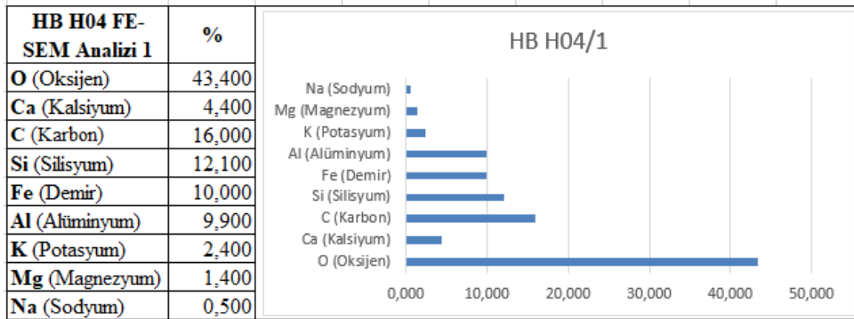
Çizelge 4.60. HB H-04/1 FE-SEM sonuçları.
