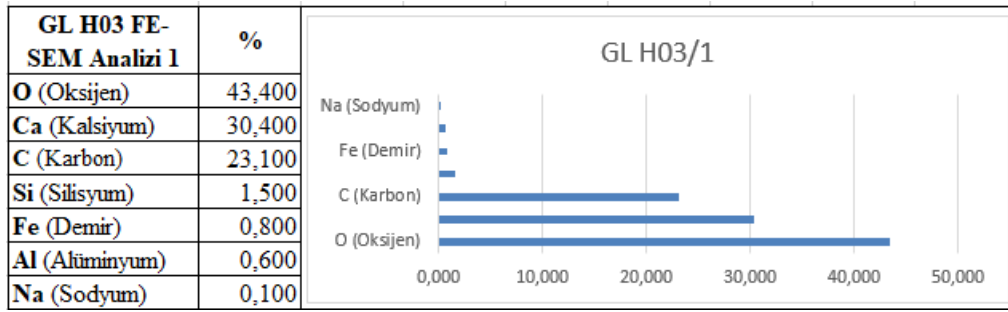
Çizelge 4.78. GL H-03/1 FE-SEM sonuçları.
