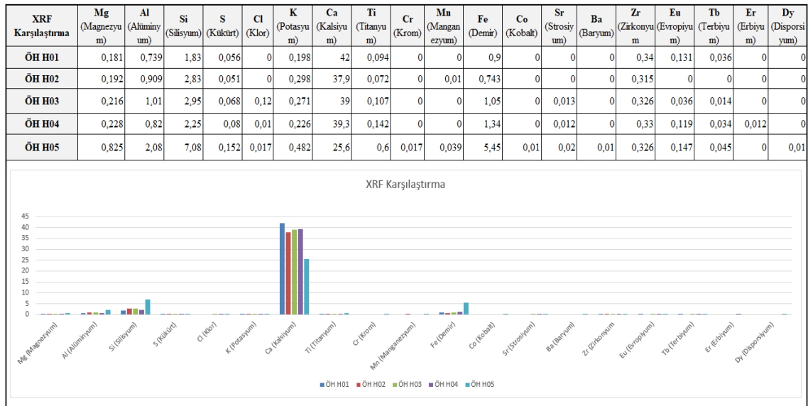
Çizelge 4.105. Öneri harçlarda XRF karşılaştırma tablosu.
