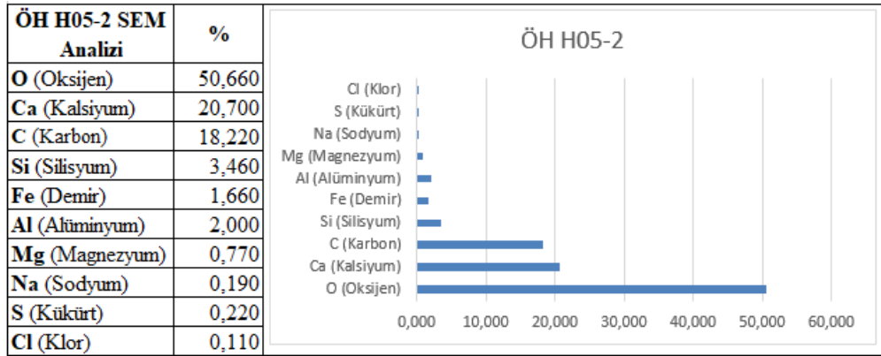
Çizelge 4.121. ÖH H-05/2 SEM sonuçları.
