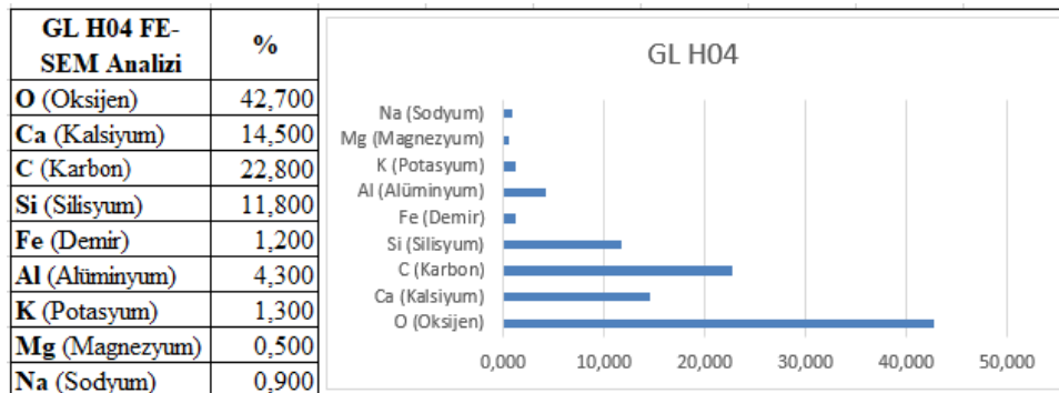
Çizelge 4.80. GL H-04 FE-SEM sonuçları.
