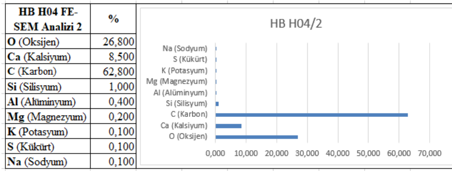
Çizelge 4.61. HB H-04/2 FE-SEM sonuçları.
