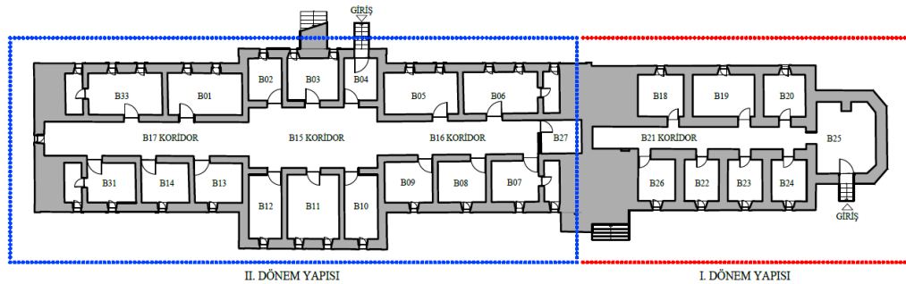
Şekil 3.10. Hemşire Lojmanı Binası rölöve projesi bodrum kat planı (DKN Mimarlık Arşivinde bulunan rölöve projesi doğrultusunda şematize edilmiştir.).
