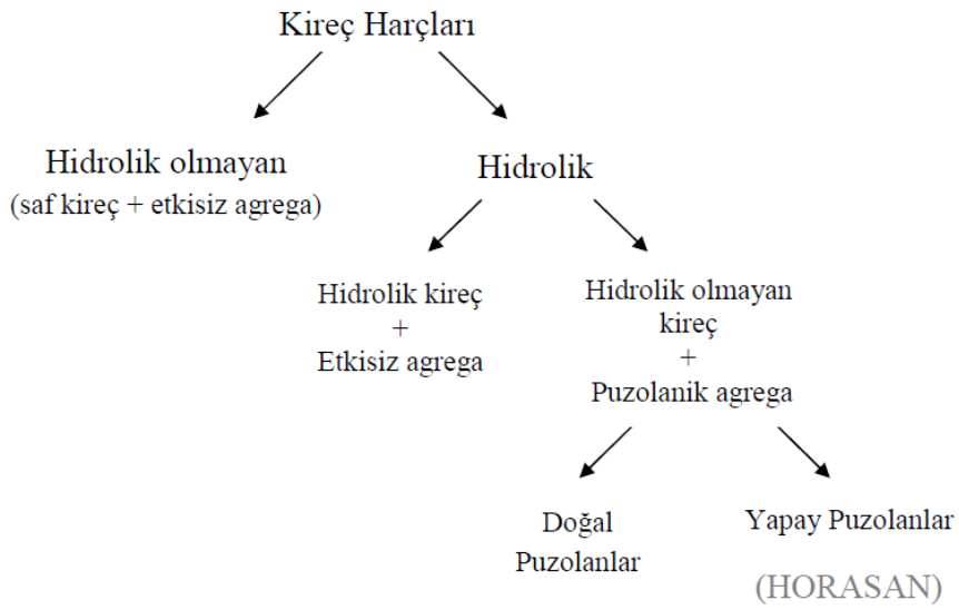
Şekil 2.9. Kireç harçların sınıflandırılması (Mavioğlu, 2011).
