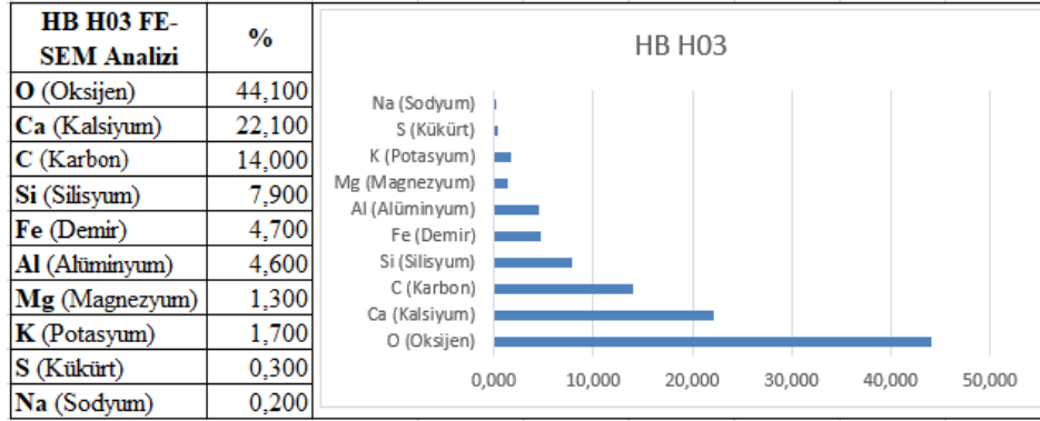
Çizelge 4.59. HB H-03 FE-SEM sonuçları.
