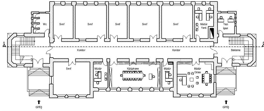
Şekil 3.56. Zemin kat planı (Parlak, 2018).
