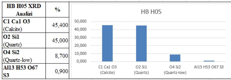
Çizelge 4.38. HB H-05 XRD sonuçları.
