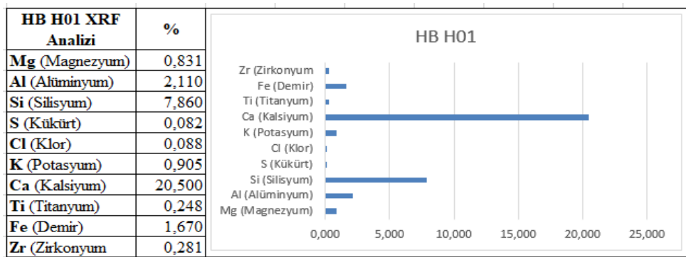
Çizelge 4.10. HB H-01 XRF sonuçları.
