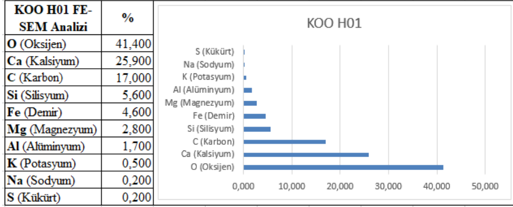
Çizelge 4.64. KOO H-01 FE-SEM sonuçları.
