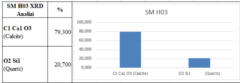
Çizelge 4.57. SM H-03 XRD sonuçları.
