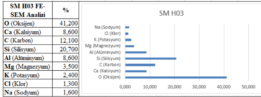
Çizelge 4.84. SM H-03 FE-SEM sonuçları.
