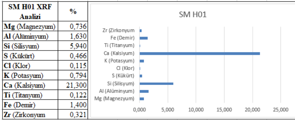
Çizelge 4.31. SM H-01 XRF sonuçları.
