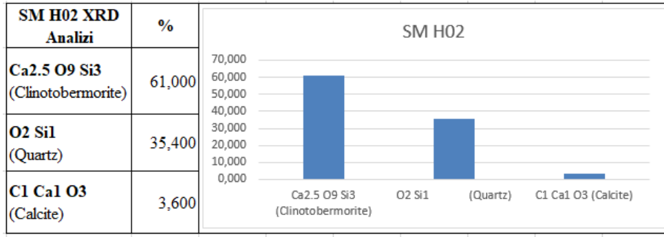
Çizelge 4.56. SM H-02 XRD sonuçları.
