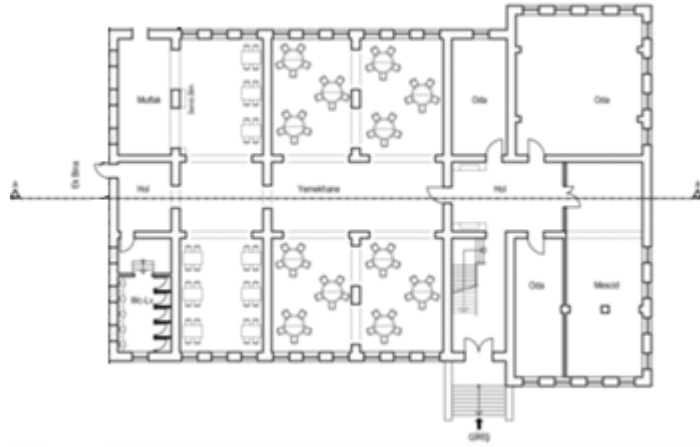
Şekil 3.25. Bodrum katı planı (Parlak, 2018).
