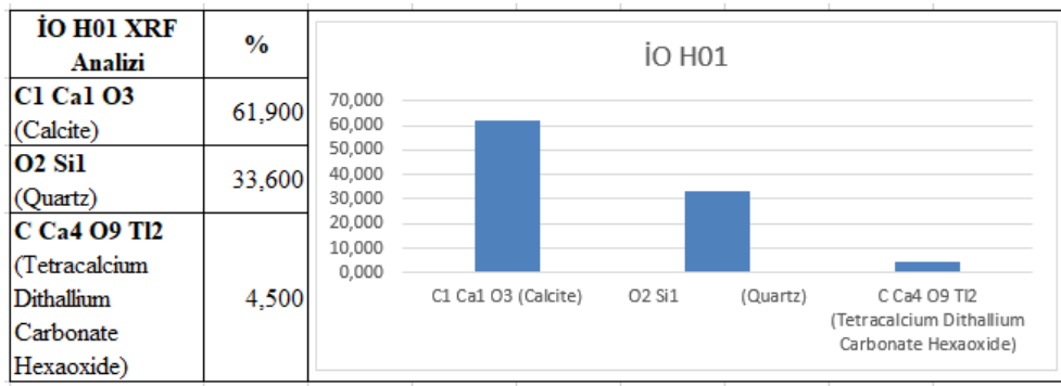
Çizelge 4.50. İO H-01 XRD sonuçları.
