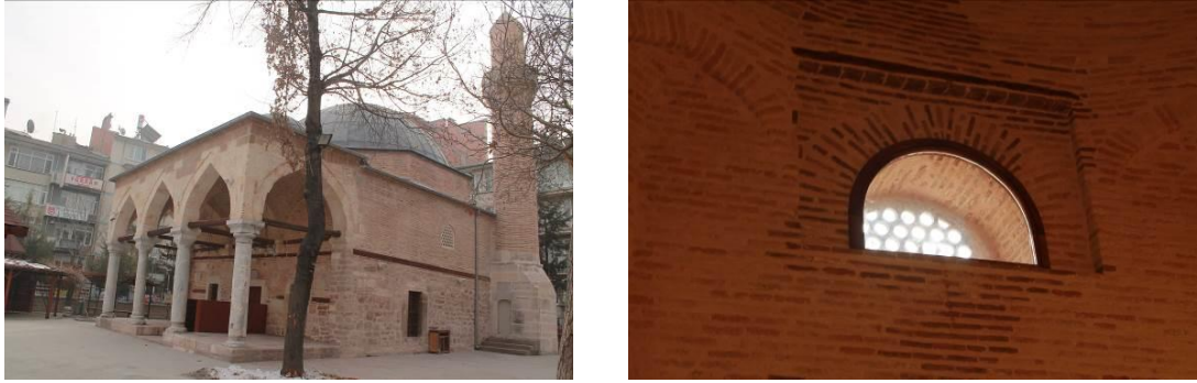
Şekil 2.19. Tuğla-taş karışık kagir duvarlı Beylikler dönemi yapısı Konya Tahir Paşa (Dursun Fakih) Camii.
