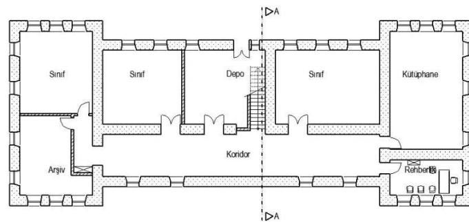
Şekil 3.48. Bodrum kat planı (Parlak, 2018).
