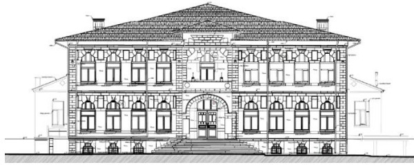
Şekil 3.23. Restorasyon öncesi yapı doğu cephe rölövesi (KUDEB Arşivi).
