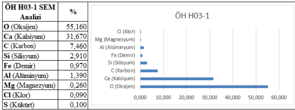
Çizelge 4.116. ÖH H-03/1 SEM sonuçları.
