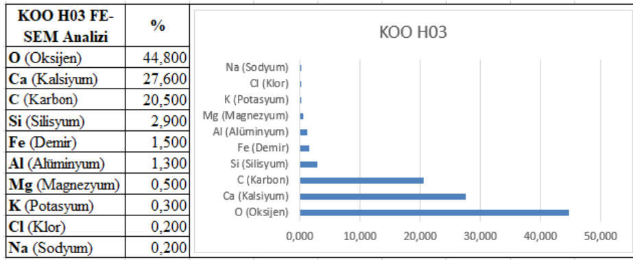
Çizelge 4.66. KOO H-03 FE-SEM sonuçları.
