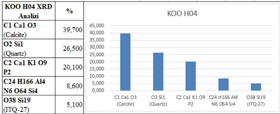
Çizelge 4.45. KOO H-04 XRD sonuçları.
