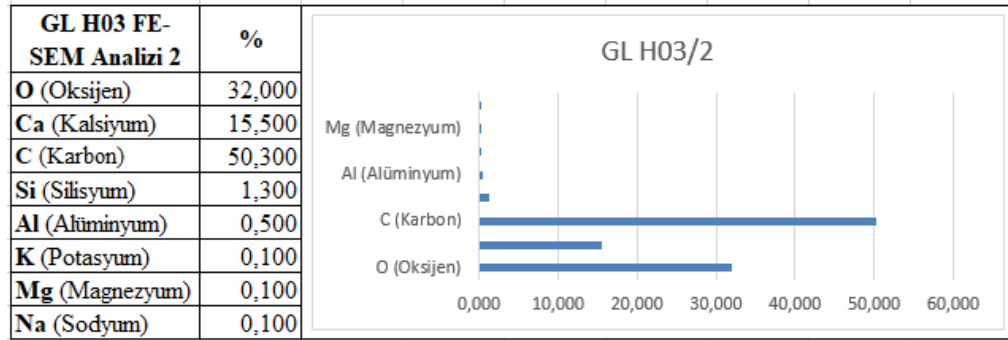
Çizelge 4.79. GL H-03/2 FE-SEM sonuçları.
