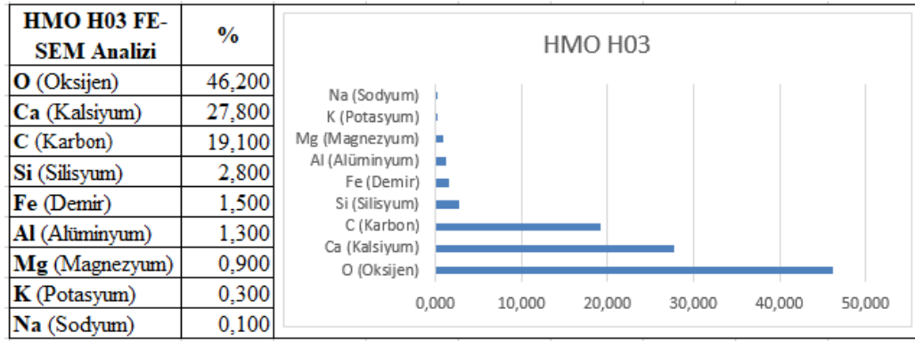
Çizelge 4.71. HMO H-03 FE-SEM sonuçları.
