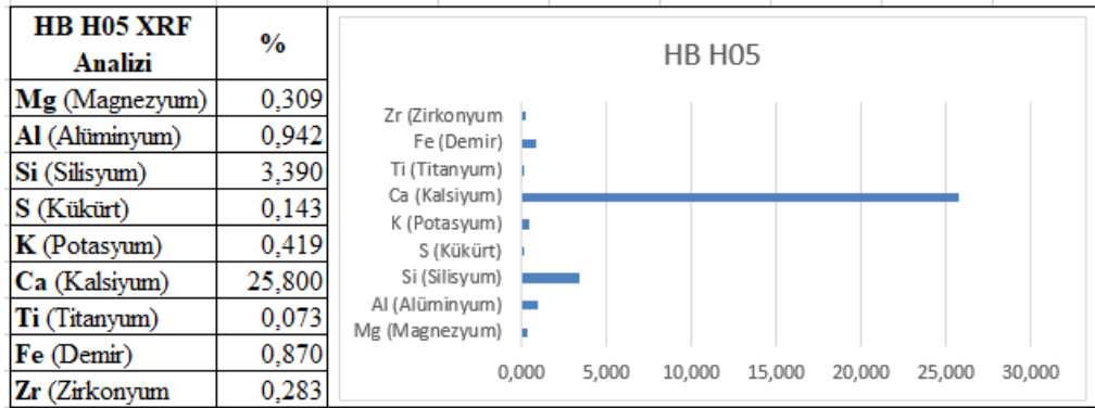
Çizelge 4.14. HB H-05 XRF sonuçları.
