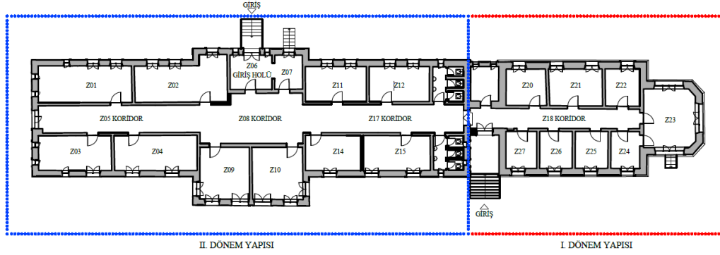
Şekil 3.9. Hemşire Lojmanı Binası rölöve projesi zemin kat planı (DKN Mimarlık Arşivinde bulunan rölöve projesi doğrultusunda şematize edilmiştir.).
