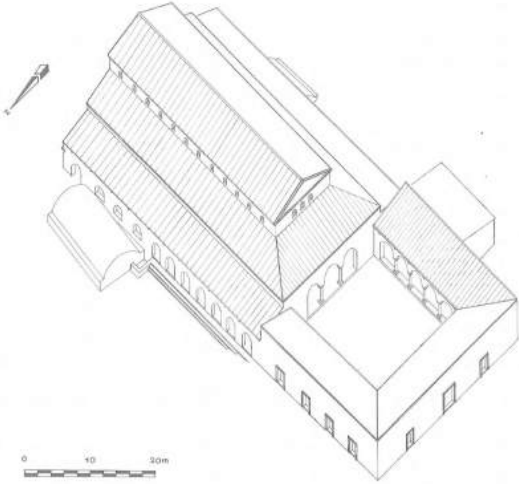
Çizim 6. Yukarı Akropol Bazilikası Restütüsüyonu (Canbilen, Lebouteiller ve Sodini, 1996: 225).
