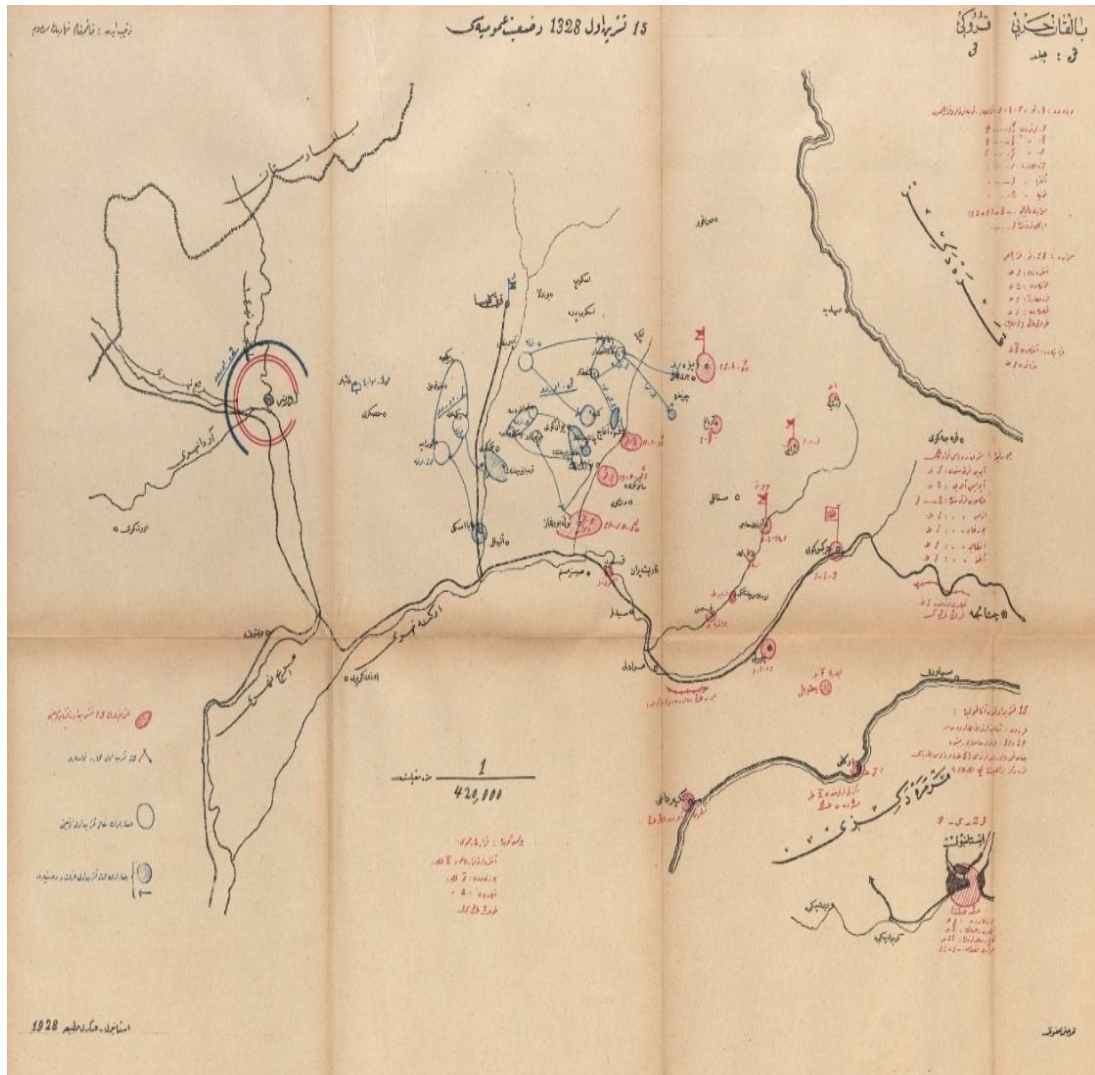
Ek 4: Karaagach Hatt'ndaki 3 numaralı tahkimat krokisi (26 Ekim 1912)
