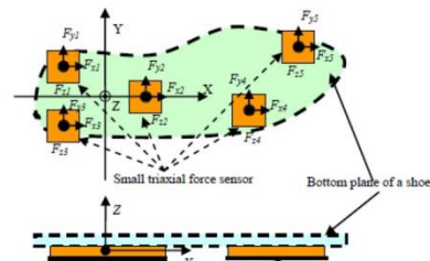
Fig 4. Insole 2
