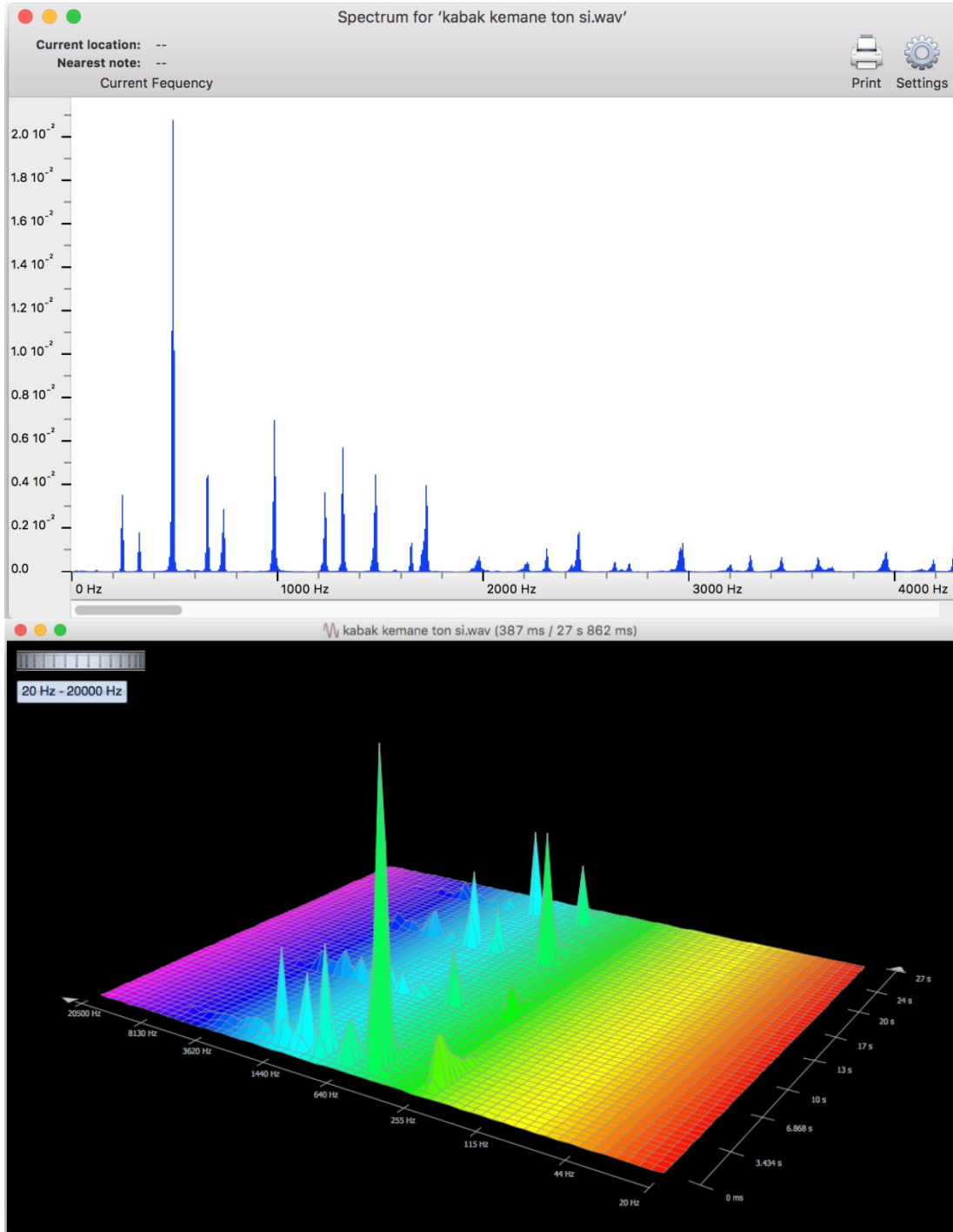
Şekil 26. Kabak Kemane Perde Frekans Analizi
