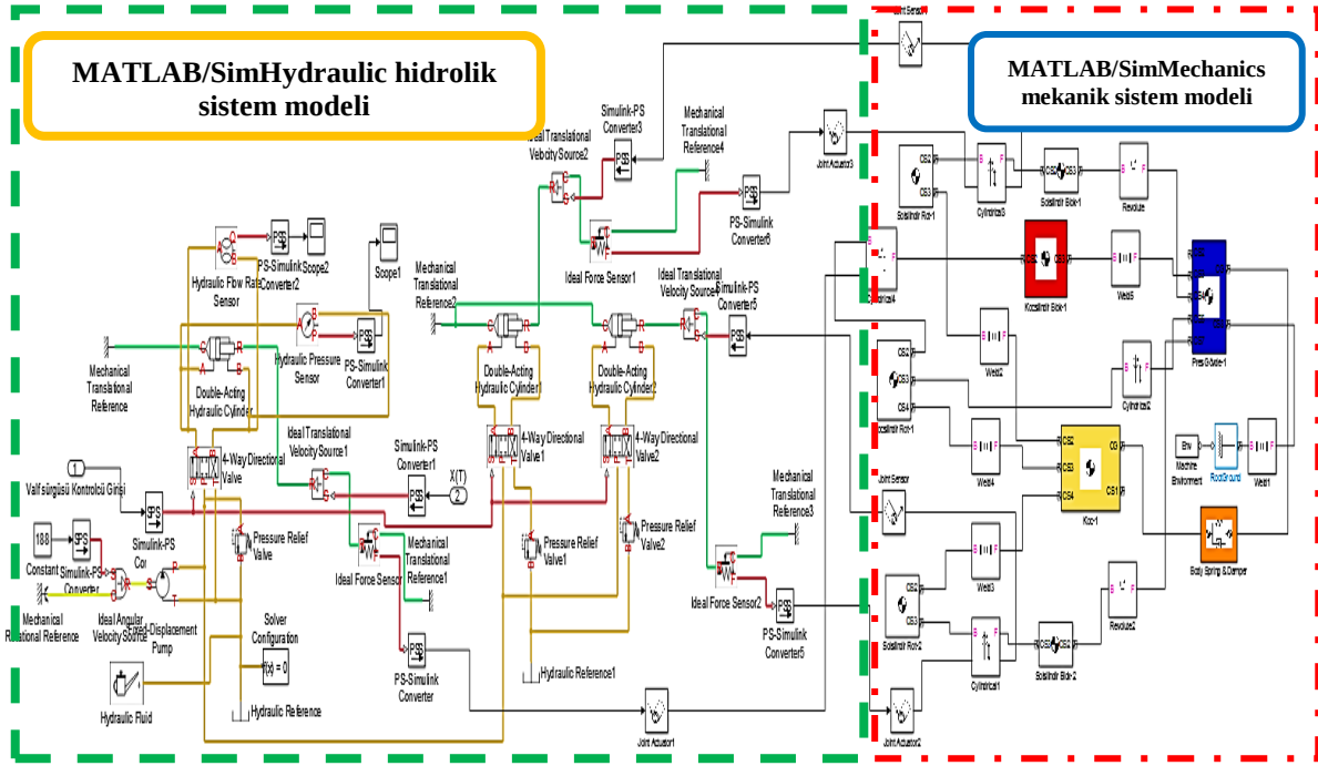
Şekil 7. MATLAB/SimMechanics ve MATLAB/SimHydraulic ile presin modellenmesi.
