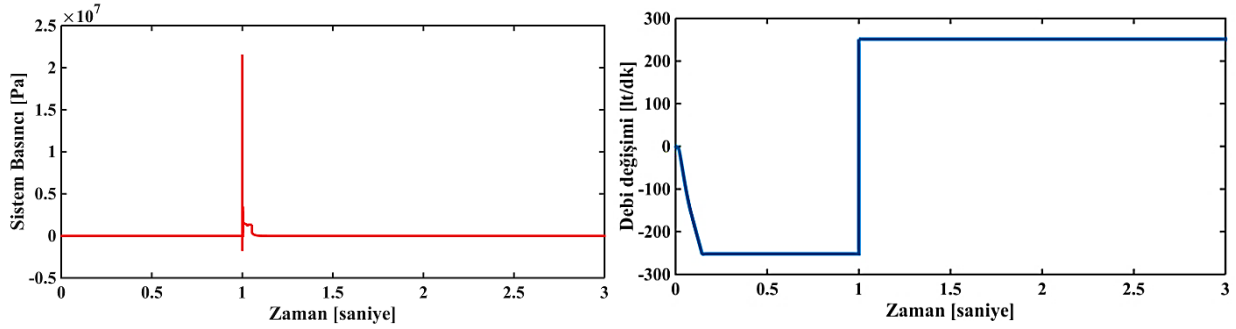
Şekil 14. Basamak giriş için elde edilen PD kontrollü basınç ve debi değişimi.
