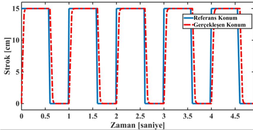
Şekil 9. Trapez giriş için elde edilen PD kontrollü strok cevabı.
