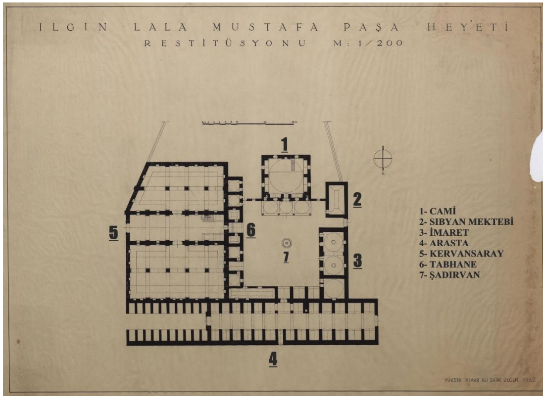
Şekil 1: Ilgın Lala Mustafa Paşa Külliyesi Planı 14
