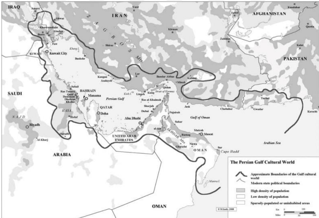
Şekil 2.3. Basra Körfezinin kültürel haritası (Potter, 2009:6)
